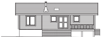
西立面図
