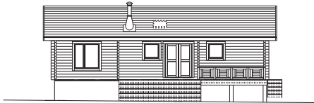
西立面図
