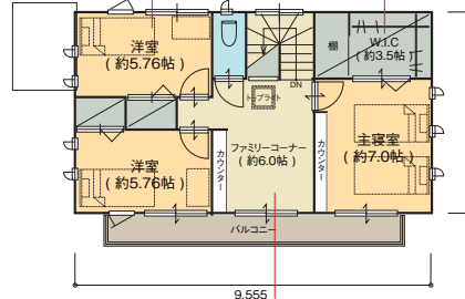
2階平面図
